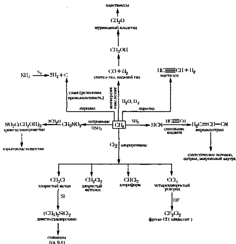
Схема 1. Промышленное использование метана
