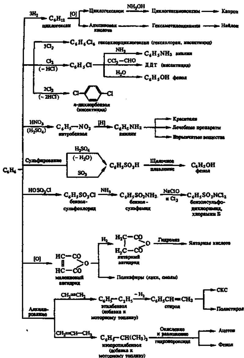
Схема 6. Промышленное использование бензола
