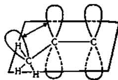
Рис. 31. Схема перекрывания орбиталей при сверхсопряжении
