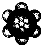
Рис. 56. Модель молекулы бензола Стюарта — Бриглеба
