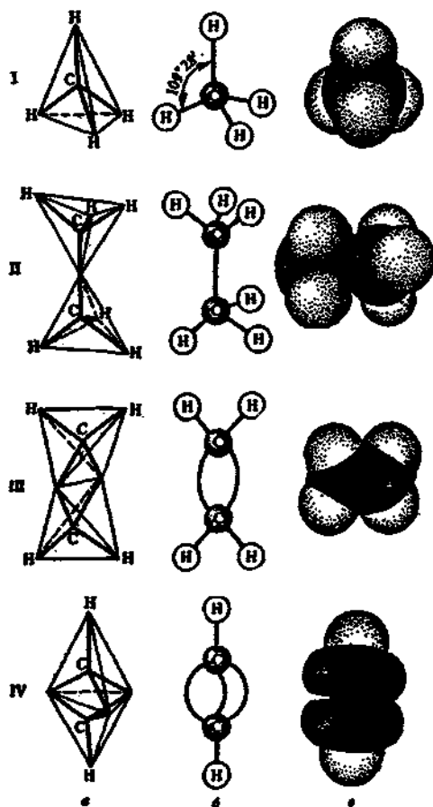
Рис. 26. Различные модели молекул метана (I), этана (II), этилена (III) и ацетилена (IV): тетраэдрические (а), стержневые (б), Стюарта — Бриггса (а)
