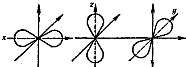
Рис. 8. Схематическое изображение электронного облака трех p -орбиталей
