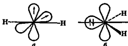
Рис. 40. Схема двух состояний карбена: триплетного (а) и синглетного
