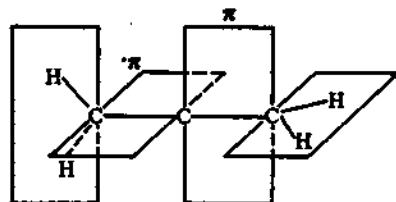
Рис. 35. Схематическое изображение строения молекулы аллена
