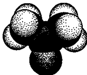
Рис. 44. Модель молекулы ацетона
