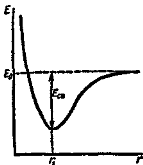
Рис. 9. Потенциальная энергия E системы как функция межъядерного расстояния r
