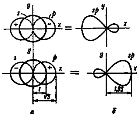
Рис. 20. Схема sp -гибридизации:
