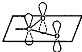
Рис. 47. Схема строения карбоксилатного иона
