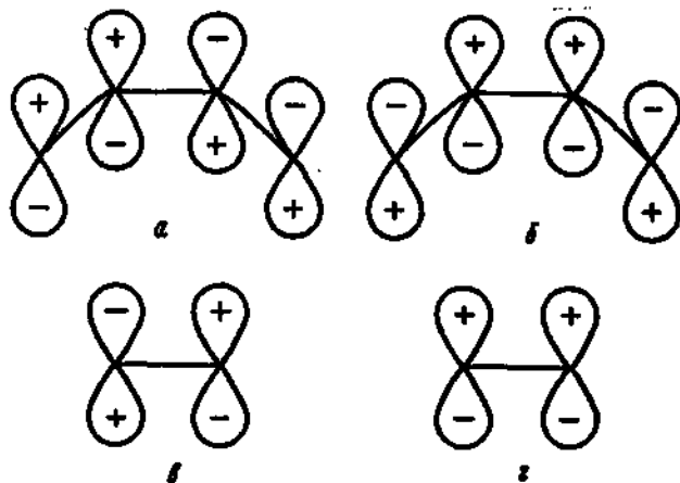
Рис. 37. Схема диенового синтеза:
