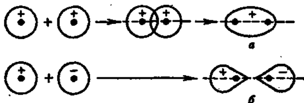
Рис. 11. Схема образования \sigma -связи при перекрывании s-орбиталей:
