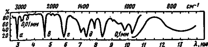
Рис. 2. Инфракрасный спектр бутинона (толщина слоя 0,01 и 0,1 мм).
