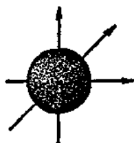
Рис. 5. Схематический вид электронного облака 1s -уровня
