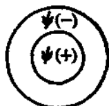
Рис. 7. Схематическое изображение электронного облака 2s -орбитали
