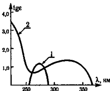
Рис. 1. Ультрафиолетовые спектры кетонов ( \varepsilon — молярный коэффициент поглощения):
